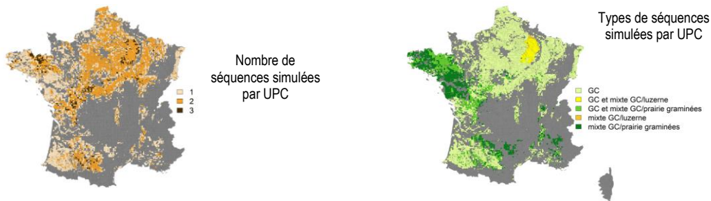
Figures 3-3. Nombre de séquences de cultures simulées par unité pédoclimatique (gauche) et types de séquences simulés (droite)
