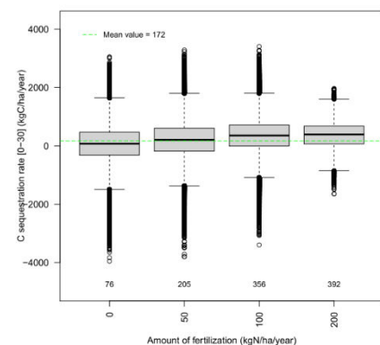
Figure 4-17. Variation moyenne annuelle absolue du stock de C (kgC/ha/an) dans l'horizon 0-30 cm des prairies permanentes productives (tous modes d'exploitation confondus) en fonction de la quantité de fertilisation azotée annuelle
